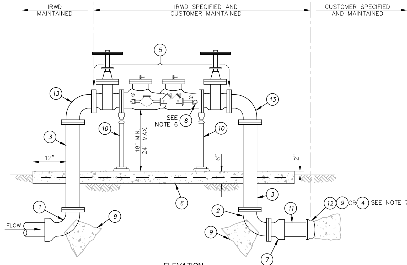
ELEVATION
