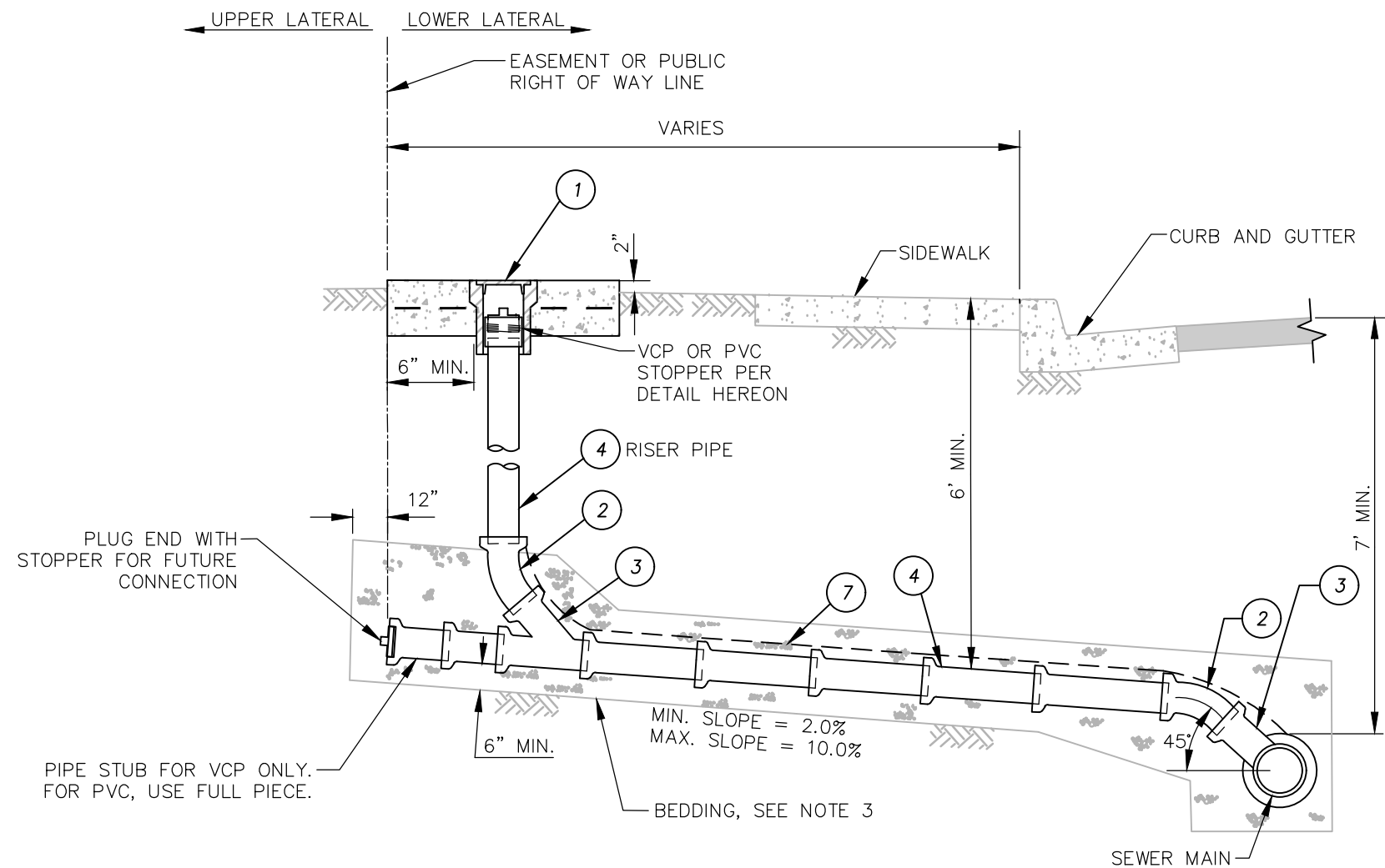
ELEVATION
