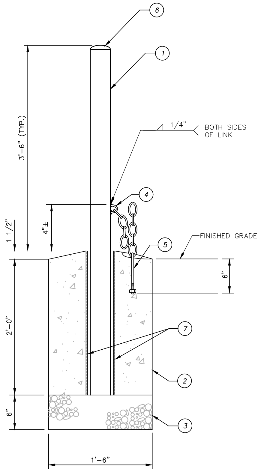
SECTION A-A
