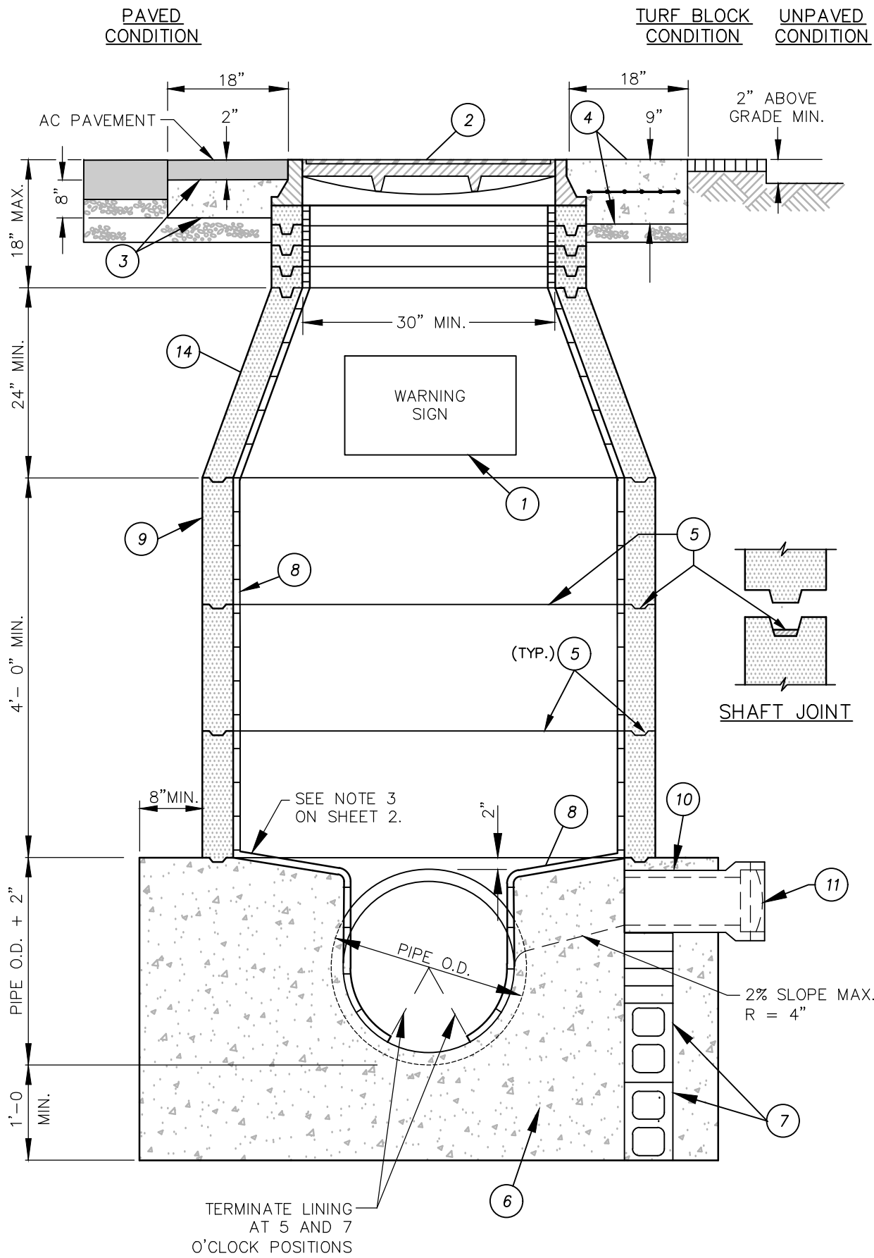
ELEVATION - MANHOLE
